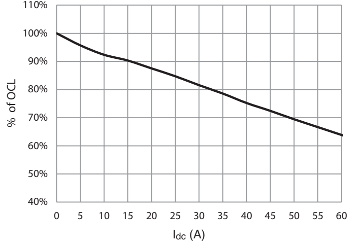
HCM1305-1R8-R
