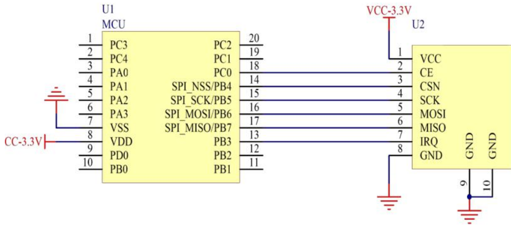
图 5-1 电路图
