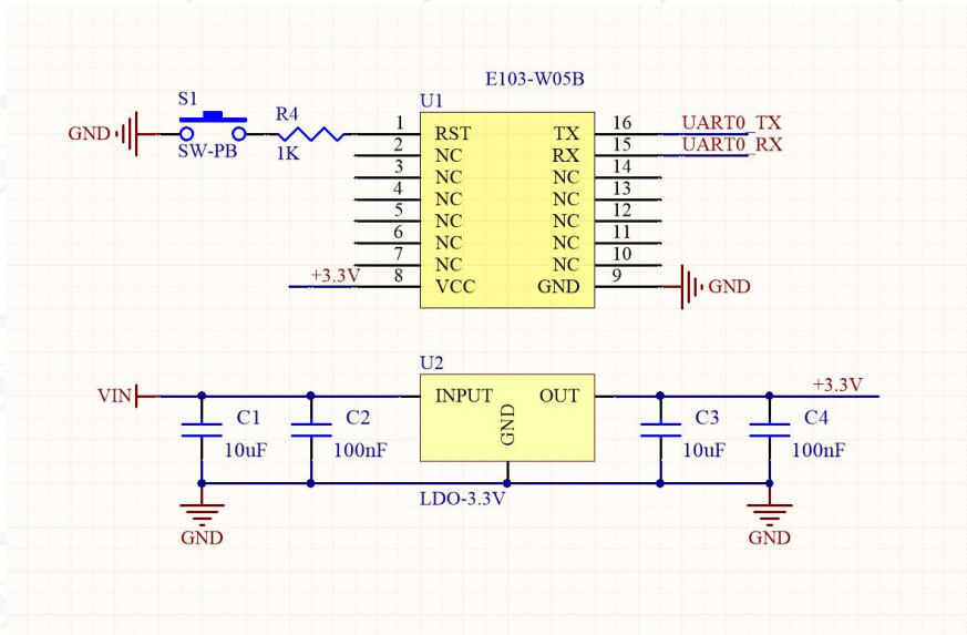
图 5-1 电路图
