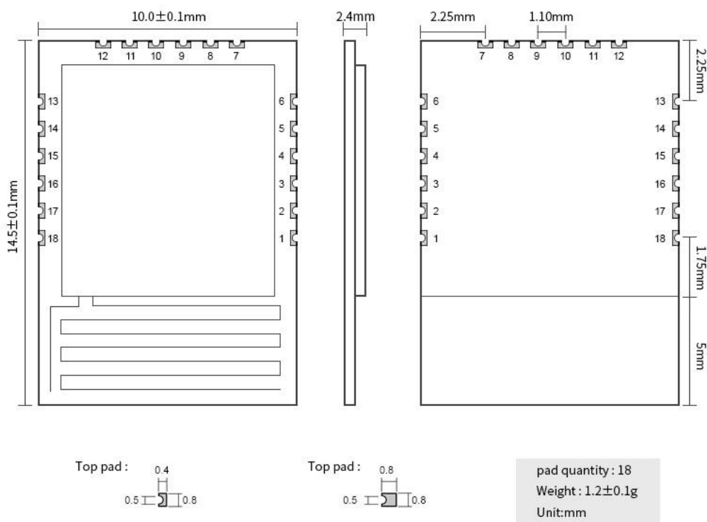
图 3-1 机械尺寸与引脚定义
