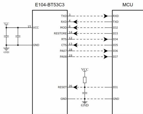
图 4-1 推荐电路
