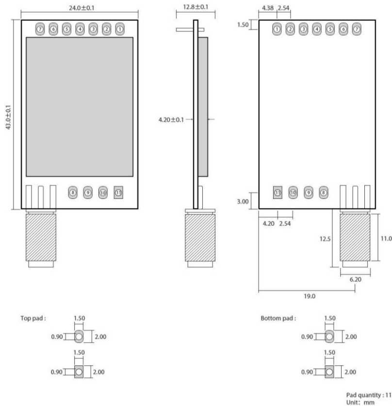
图 3-1 机械尺寸与引脚定义
