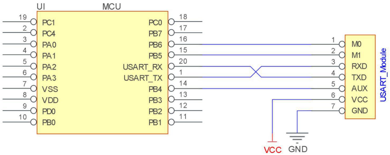
图 4-1 推荐连线图
