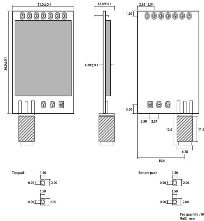
图 3-1 机械尺寸与引脚定义
