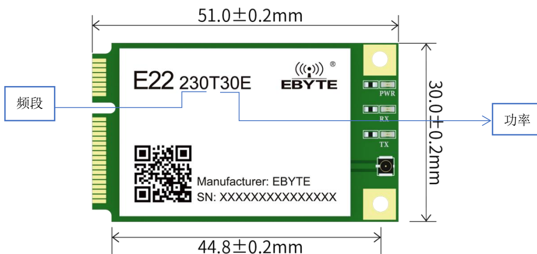
注：上图为 E22-230T30E 模块的 3D 尺寸图，其余模块与它尺寸一致，引脚兼容，频段和功率不同。
