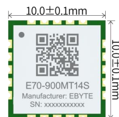
图 4: E70-900MT14S
