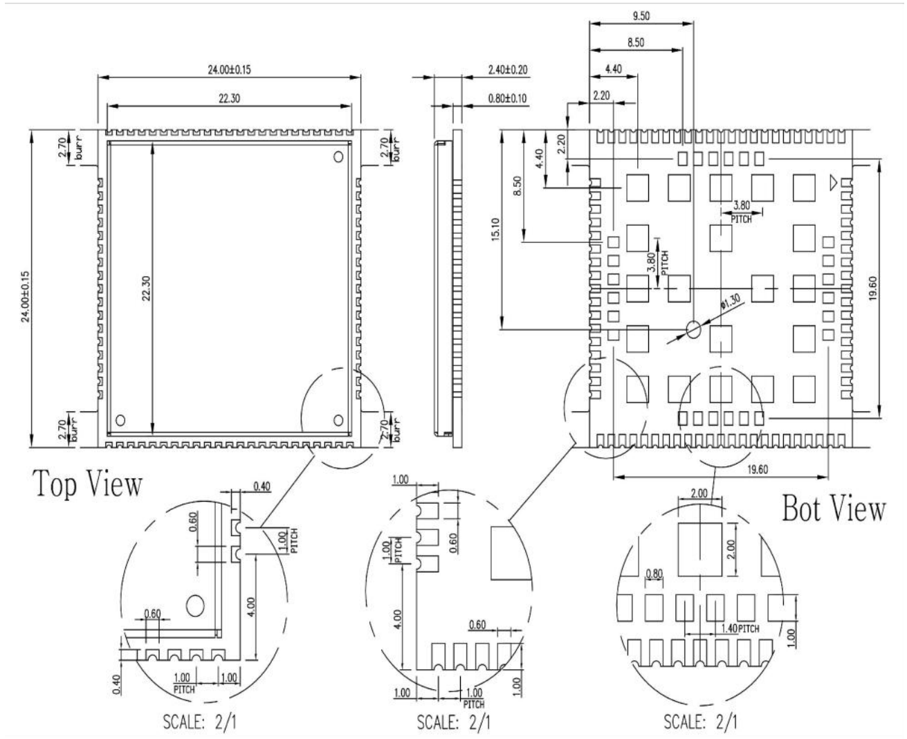
模块尺寸图 (单位：毫米)
