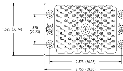
120 PIN RECEPTACLE
