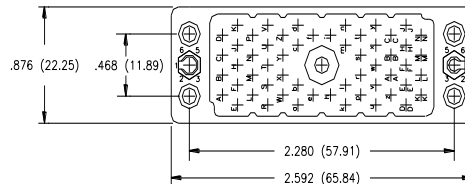
56 PIN RECEPTACLE
