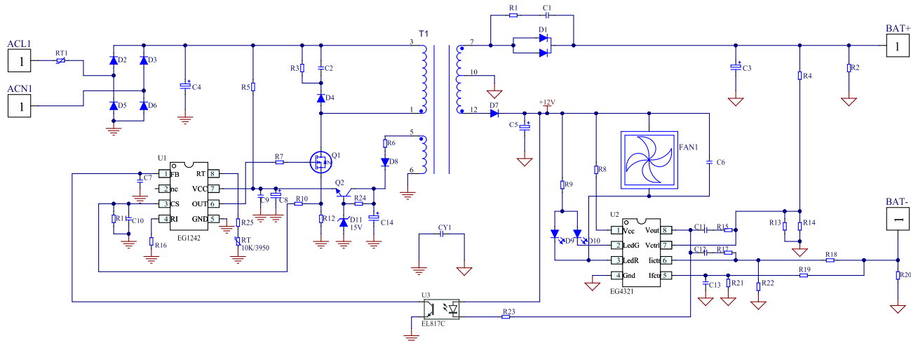
图 6-3. EG1242+EG4321 宽电压范围恒压恒流锂电池充电器应用图
