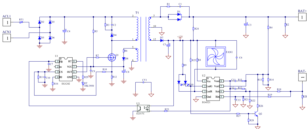
图 6-2. EG1242+EG4321 三段式铅酸电池充电器应用图
