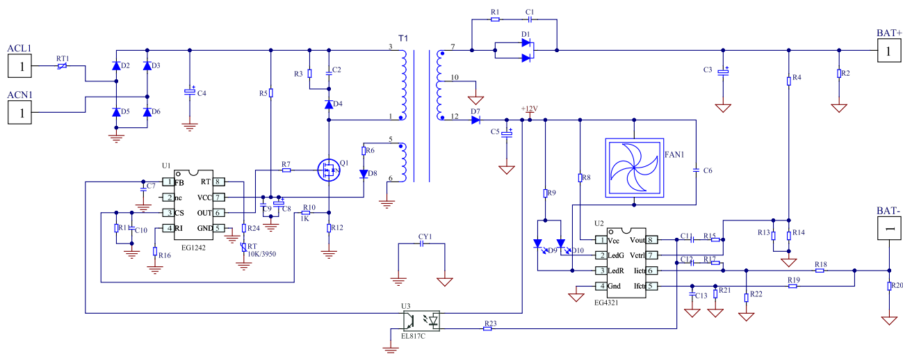
图 6-1. EG1242+EG4321 恒压恒流锂电池充电器应用图
