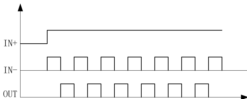
图7-3. 反向驱动
