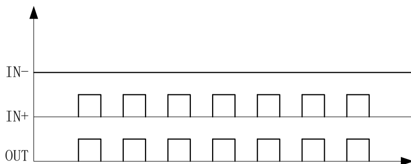
图7-2. 同向驱动
