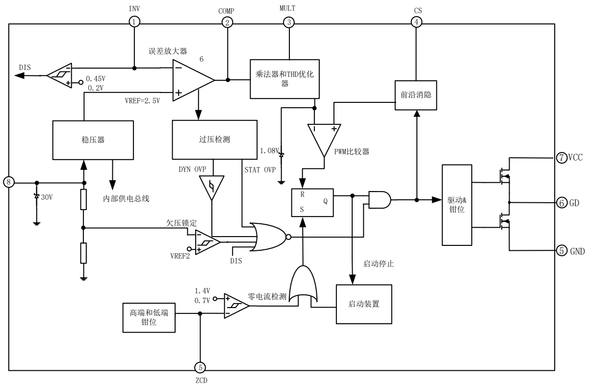
图 5-1. EG6562 结构框图
