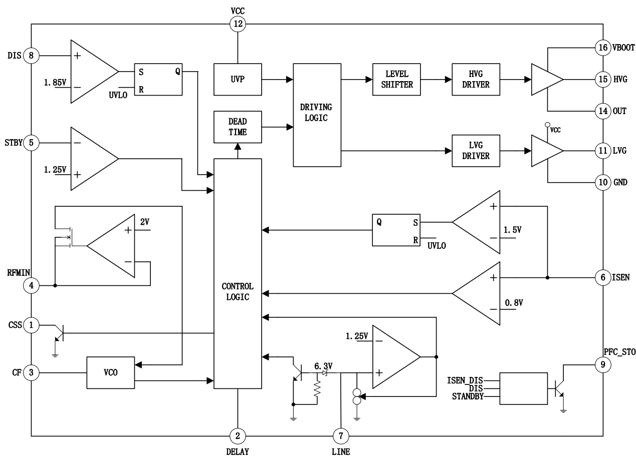
图5-1. EG6599内部电路图
