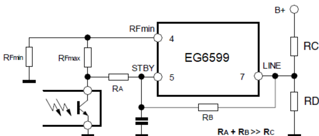
图 8-5 宽输入电压时的猝发工作模式
