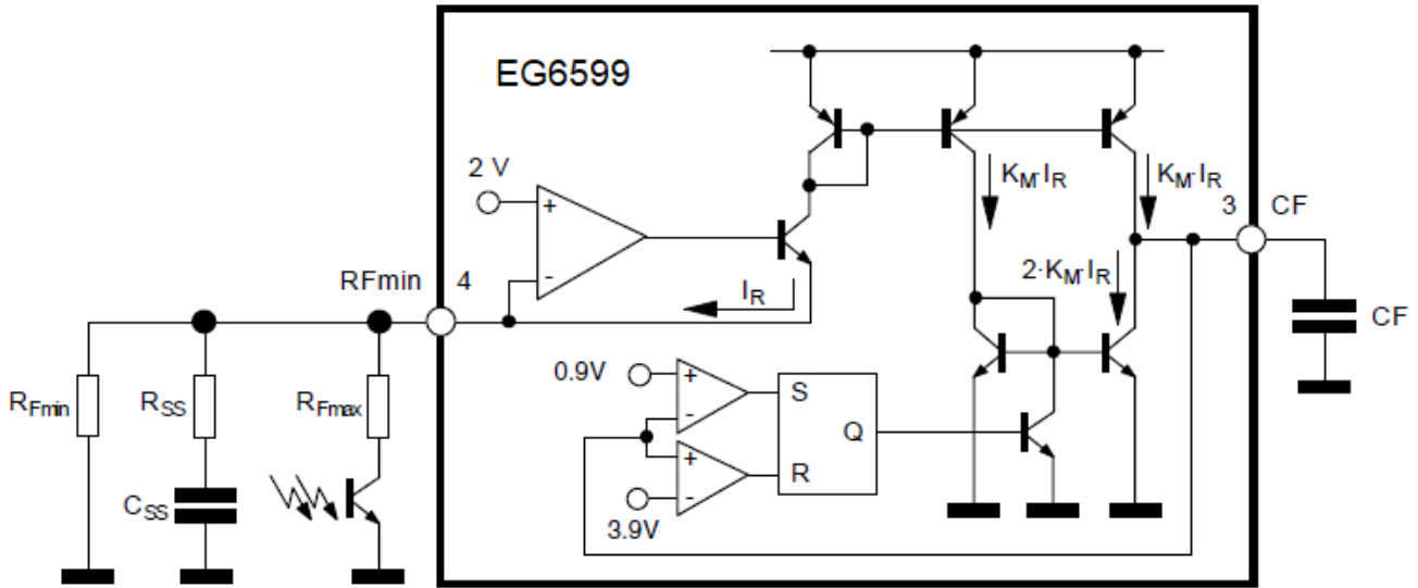
图8-2. 振荡器框图
