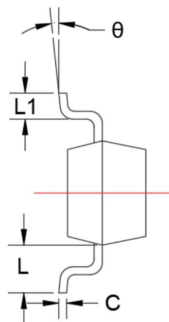
SOT-23
