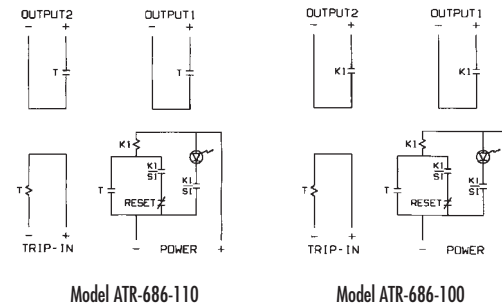
WIRING SCHEMATICS
