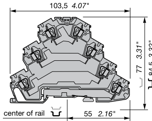
D 2,5/5.T3.PL
