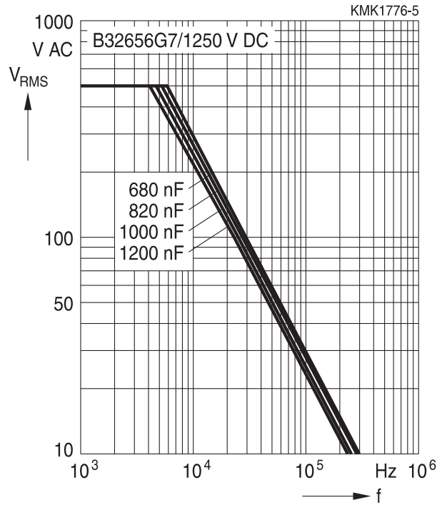
1250 V DC/500 V AC, B32656G7
