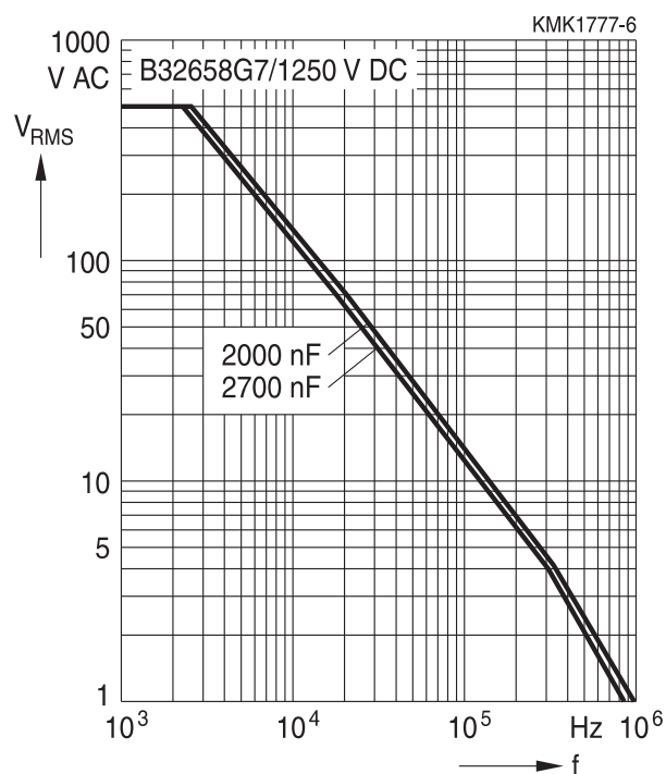
1250 V DC/500 V AC, B32658G7
