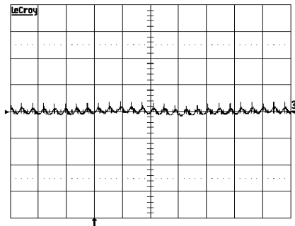
Trace: output voltage (10 mV/div.). Time scale: (5 \mu\text{s} /div.).
