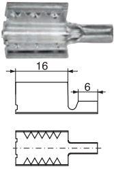
Końcówka typ TEL 2,5 (do łączników ekranu O)
