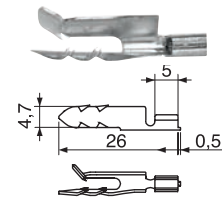
Końcówka typ EL 1,5 (do łączników ekranu A)
