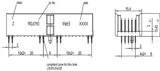
compliant zone for thru hole DIN 6750
