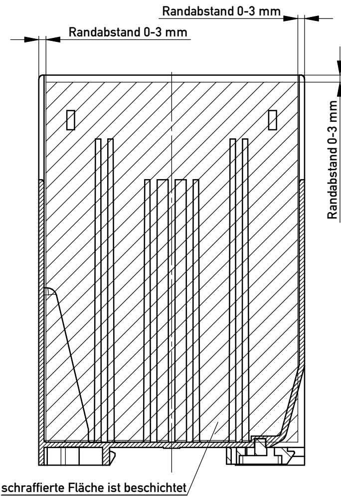
SCHNITT B-B
