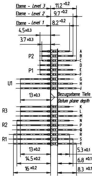
Lochbild für Leiterplatte (Bestückungsseite) für Einpresstechnik
