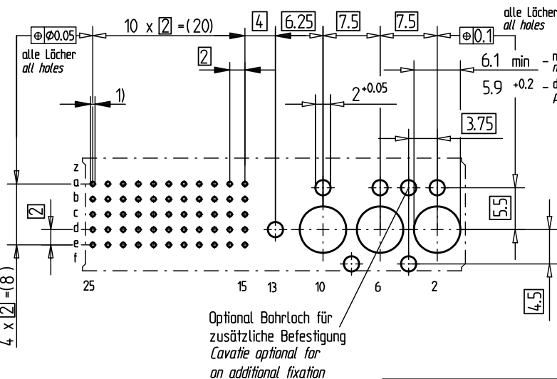
Lochbild für Leiterplatte (Bestückungsseite)
