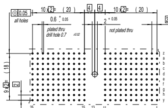
Lochbild fuer Leiterplatte (Bestückungsseite)
