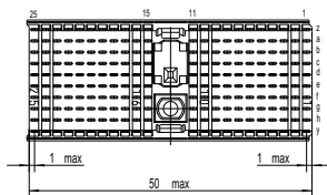
Lochbild fuer Leiterplatte (Bestückungsseite)
