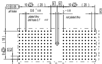
Lochbild fuer Leiterplatte (Bestückungsseite)
