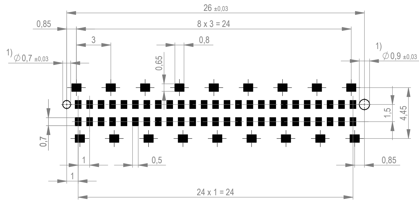
1) Durchmesser des Bohrers / drill tool
