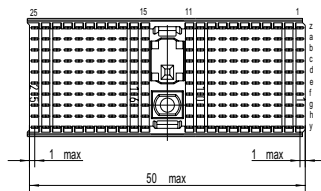
Lochbild fuer Leiterplatte (Bestückungssseite) Board hole pattern (Component mounting side)
