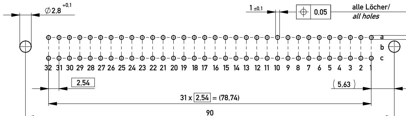
Leiterplatten-Lochbild / PCB drillhole Pattern
