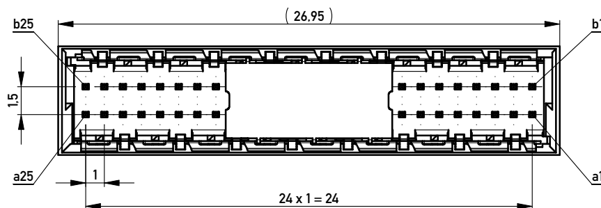
Leiterplatten-Layout Vorschlag / PCP-Layout Proposal
