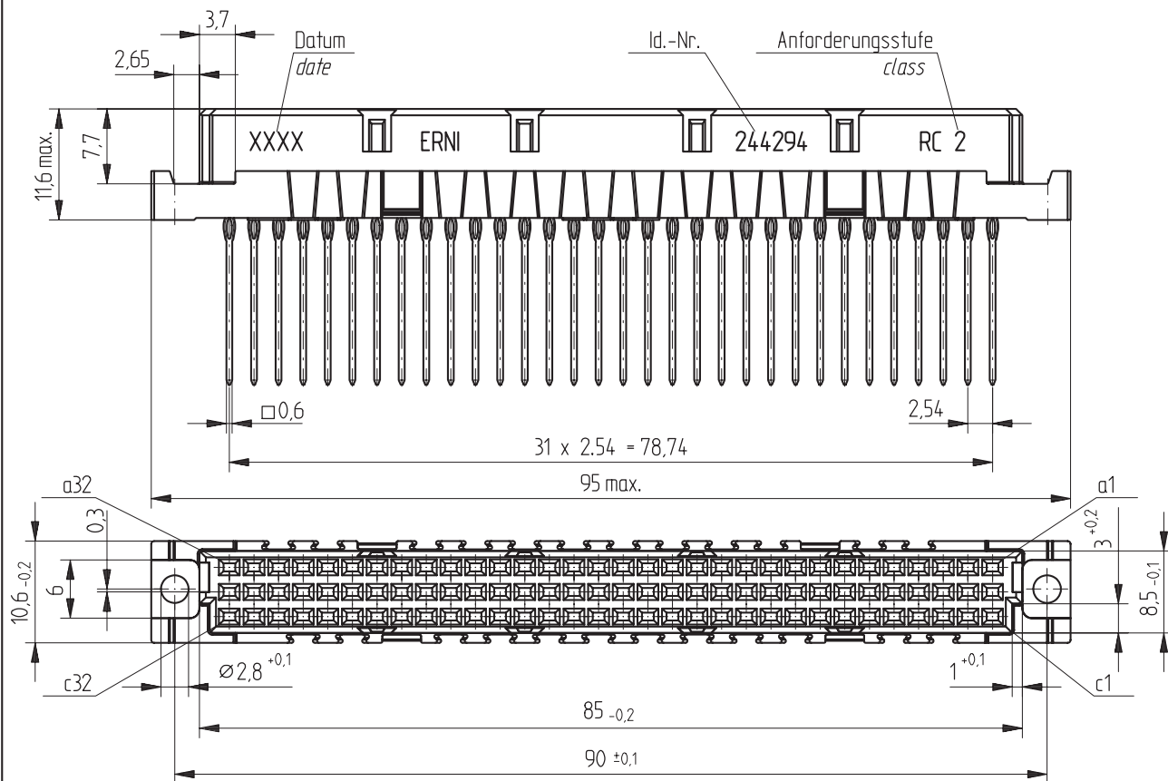
Bestückungsplan / contact layout ■ bestückt / assembled
