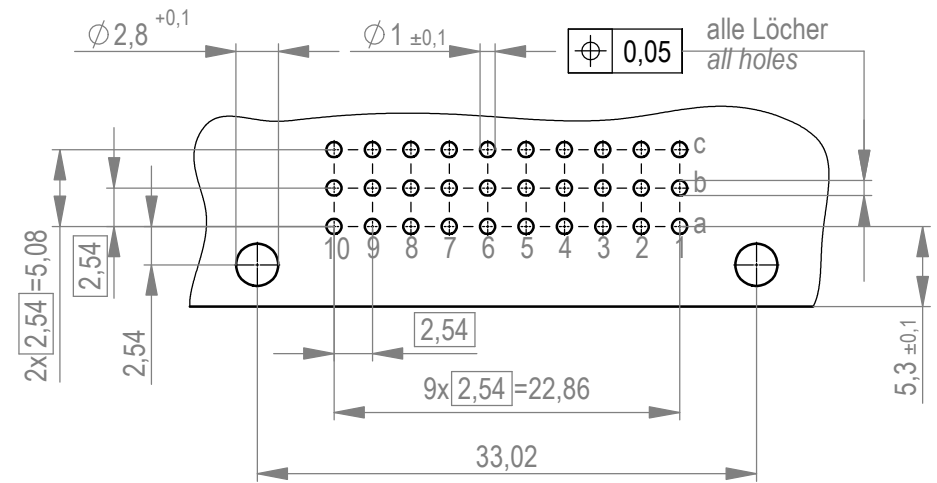
Leiterplatten- Lochbild / PCB drillhole pattern
