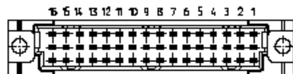
Leiterplatten-Lochbild / PCB drillhole pattern
