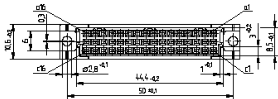
Bestückungsplan / contact layout ■ bestückt / assemble
