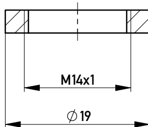
Schnitt A-A
