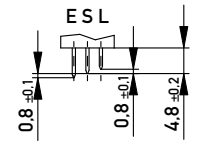
Stecklänge / mating length
