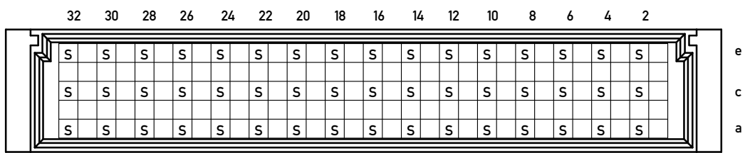
Leiterplatten-Lochbild / PCB drillhole pattern
