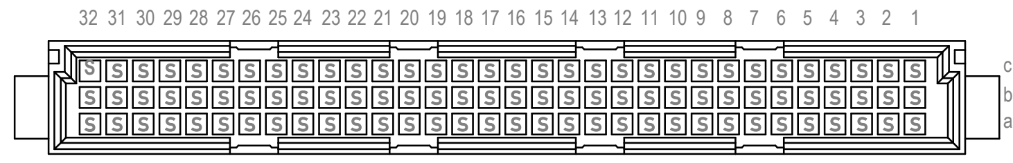
Leiterplatten-Lochbild / PCB drillhole pattern
