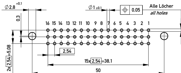
Leiterplatten-Lochbild / PCB drillhole pattern
