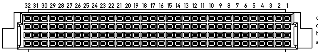
Bestückungsplan / contact layout
