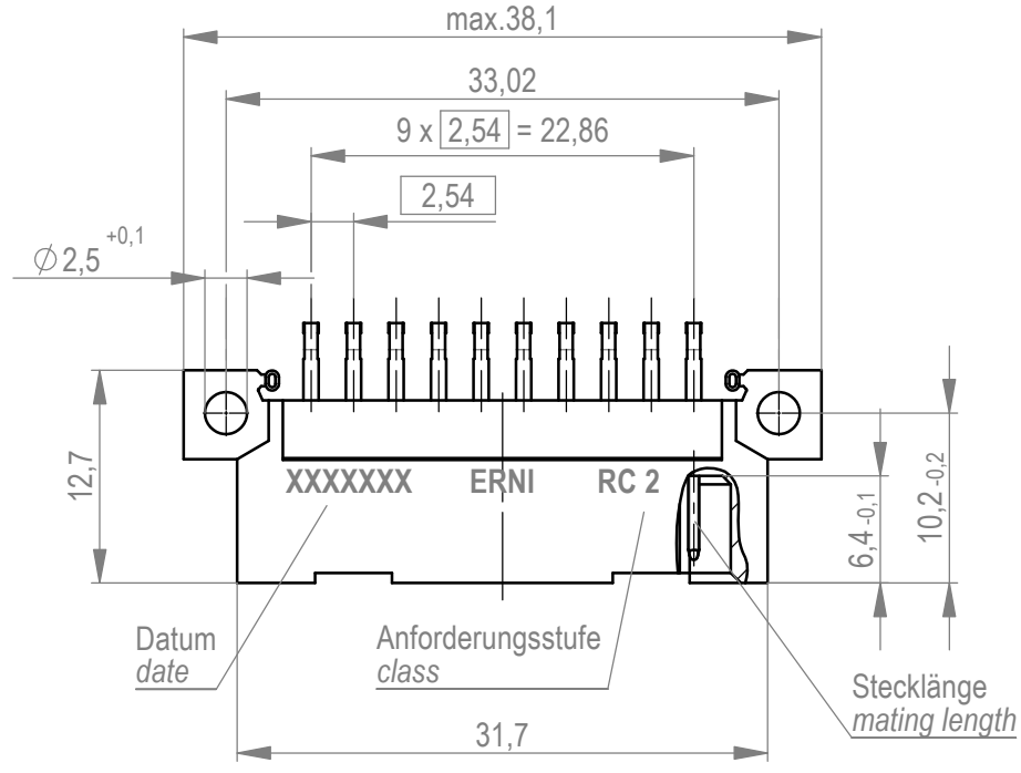
Bestückungsplan / contact layout
