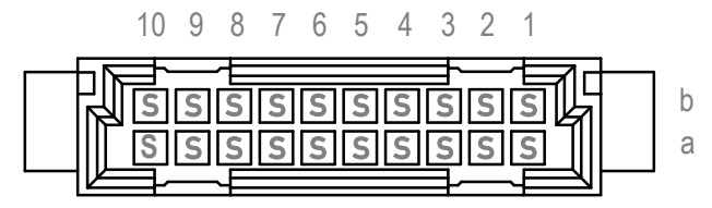
Bestückungsplan / contact layout
