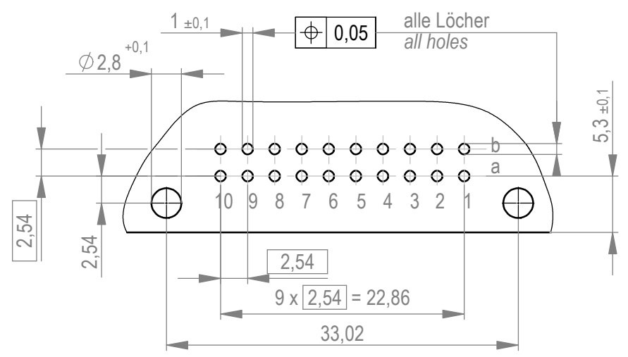
Leiterplatten- Lochbild / PCB drillhole pattern
