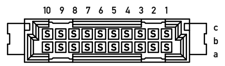
Leiterplatten- Lochbild / PCB drillhole pattern
