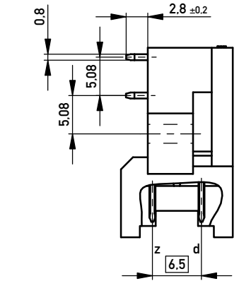
Bestückungsplan / contact layout
