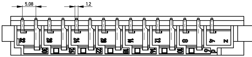
Bestückungsplan / contact layout
