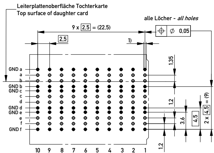
Lochbild für Leiterplatte PCB drill hole pattern (Sicht auf Bestückungsseite) (Component mounting side)
