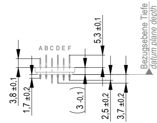
Kontaktversionen, Messerkontakte contact selection options, male contacts
