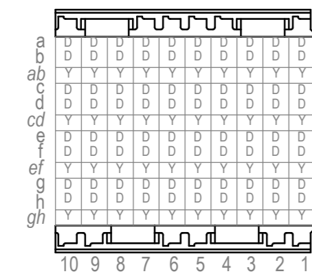
Bestückungsplan - contact layout
