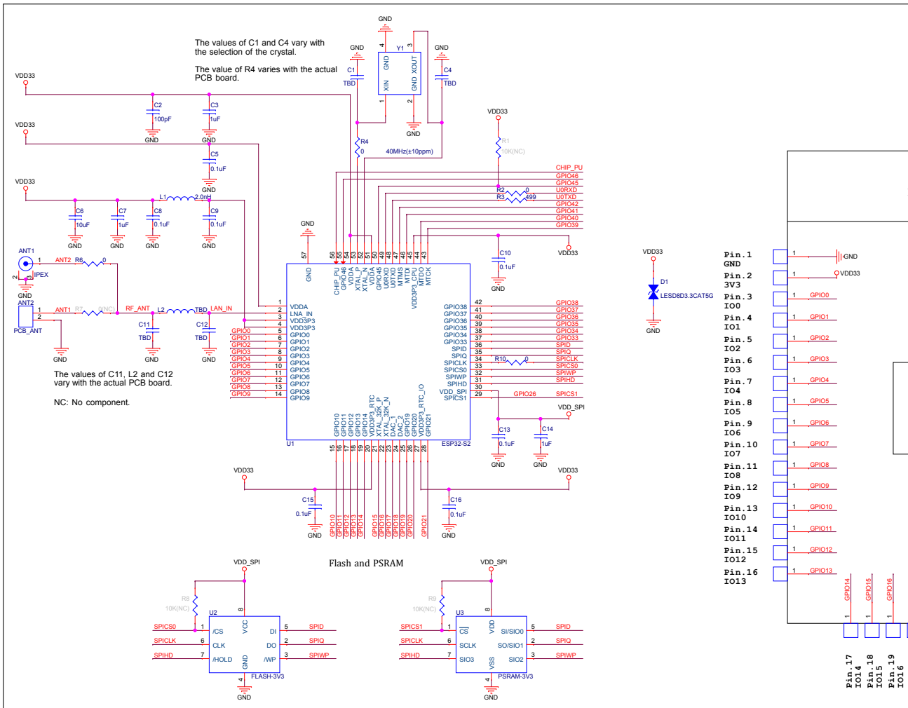
图 5: ESP32-S2-WROVER-I 原理图
