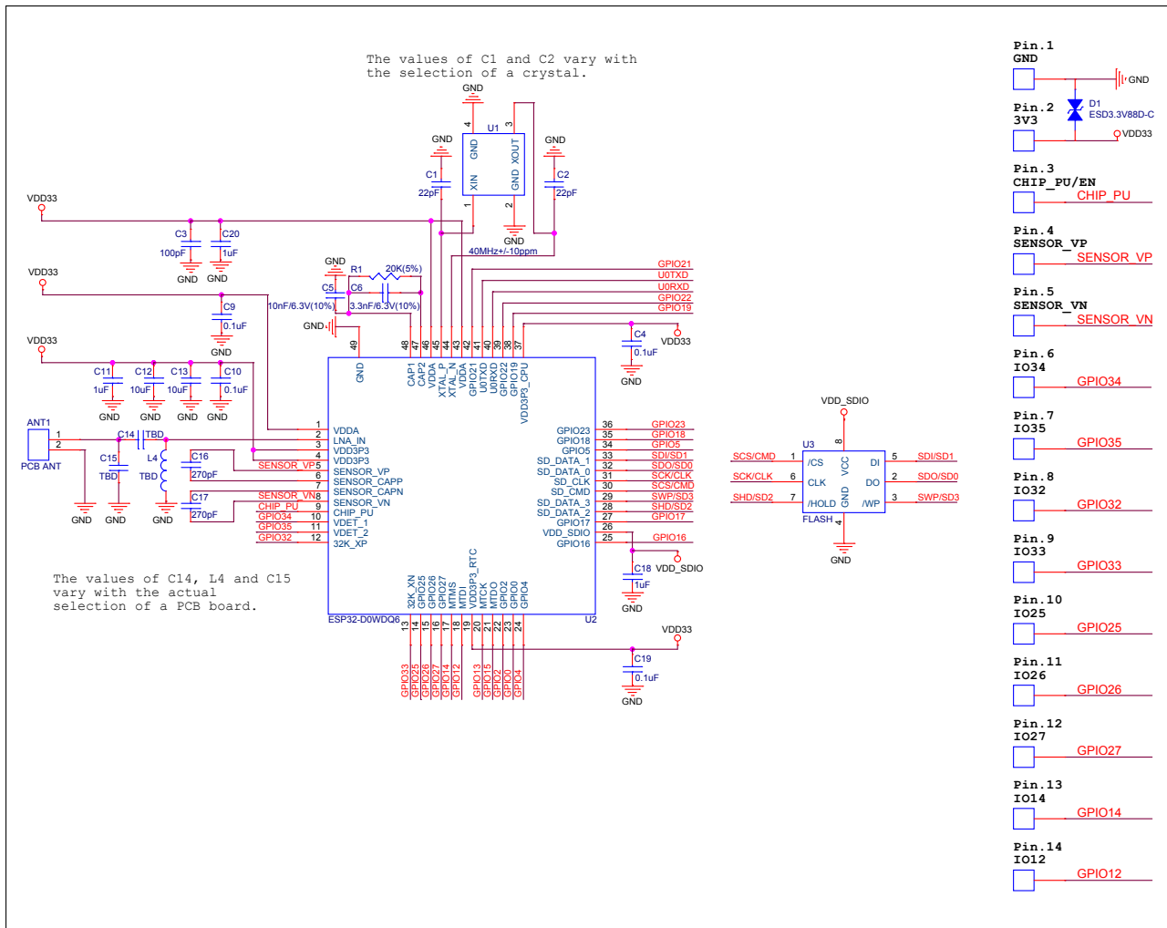
图 3: ESP32-WROOM-32 电路原理图
