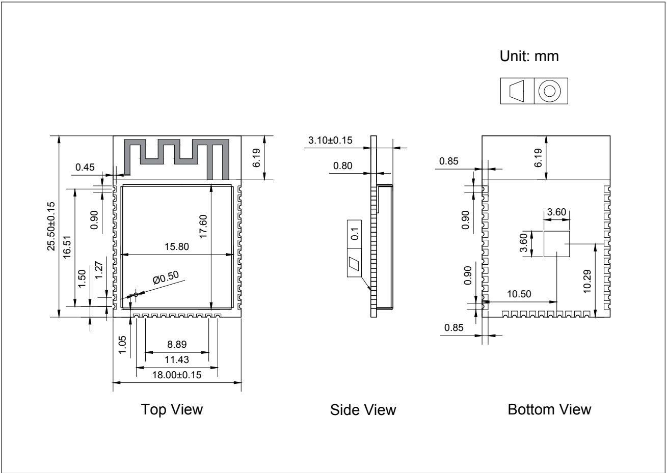
图 6: ESP32-WROOM-32D 尺寸
