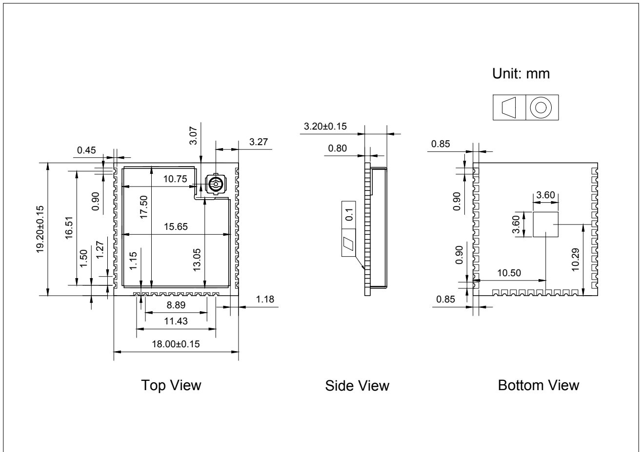
图 7: ESP32-WROOM-32U 尺寸
