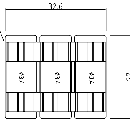
EFA04 71 P02 \phi 3.4 COUPLER CLIP
