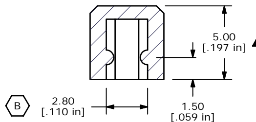
SECTION A-A SCALE 4 : 1
